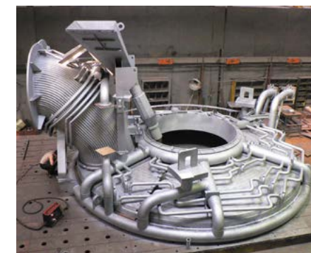
Свод в сборе печи ДСП
